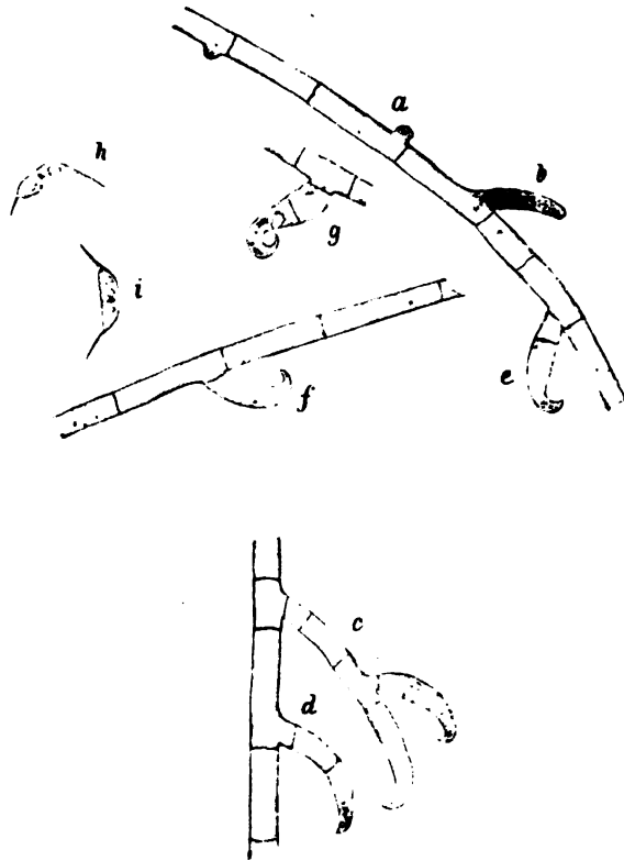
Fig. 1. Eriouema ciliatum . 600/1.
